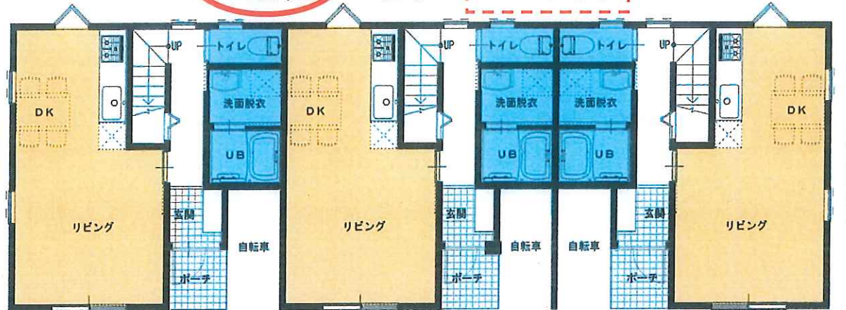
一階間取図
